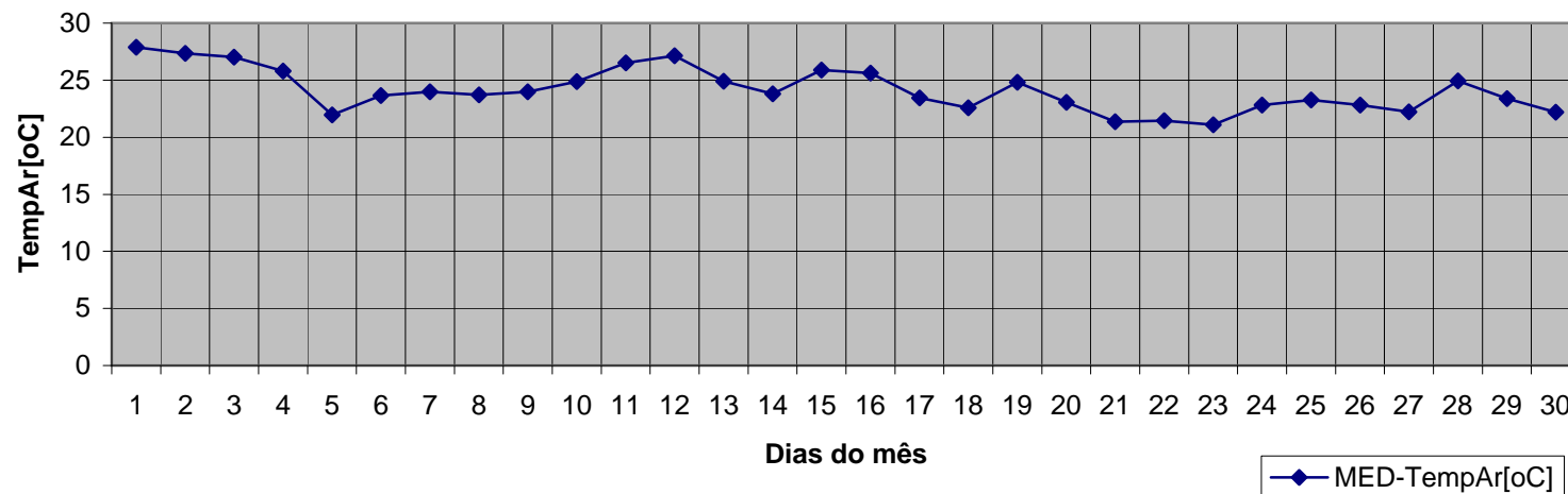
Média temperaturado ar de novembro_2007
