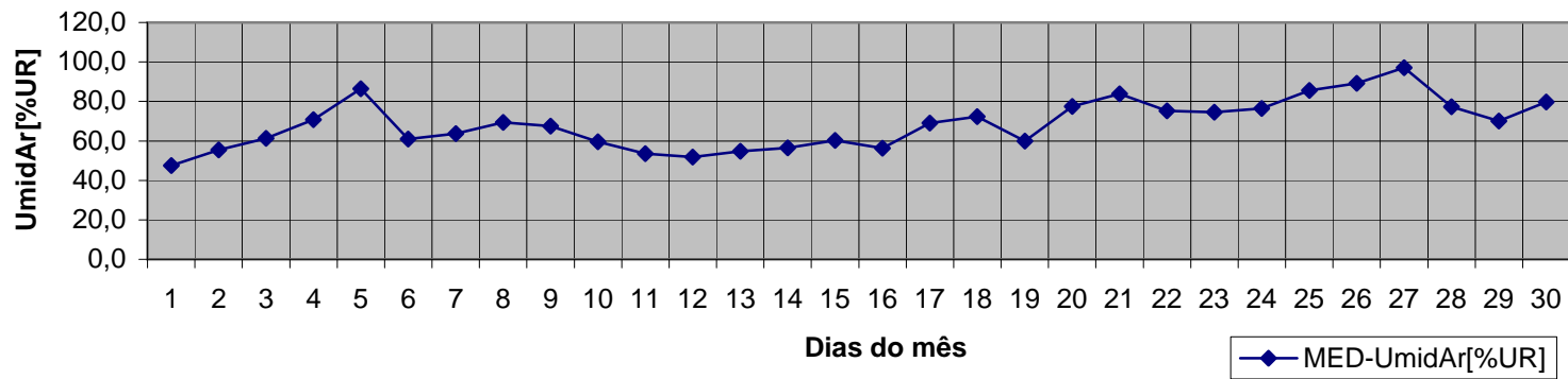
Médiada umidade relativa do ar de novembro_2007
