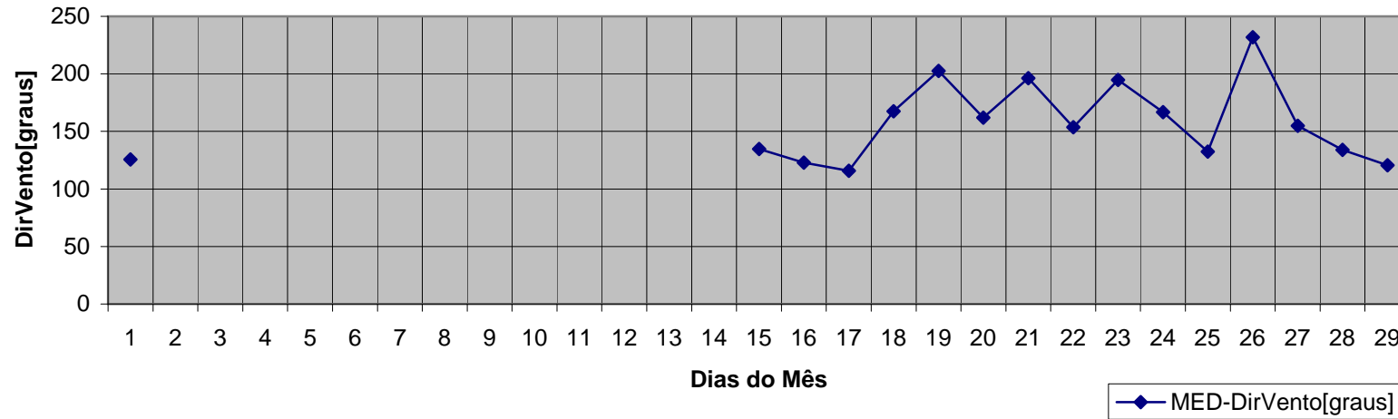
Média da direção do vento de fevereiro_2008
