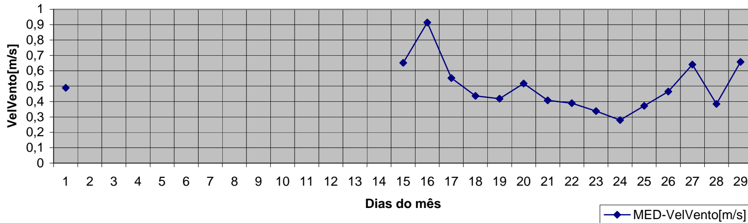
Média velocidade do vento de fevereiro_2008
