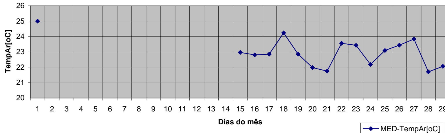
Média da temperatura de fevereiro_2008
