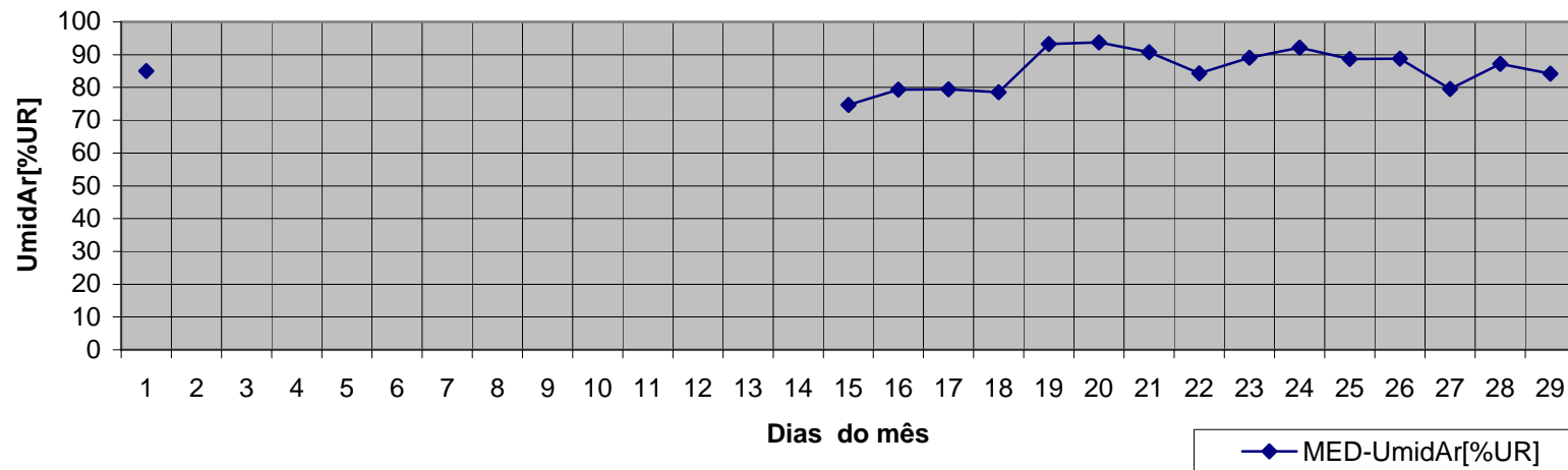
Média da umidade relativa do ar de fevereiro_2008
