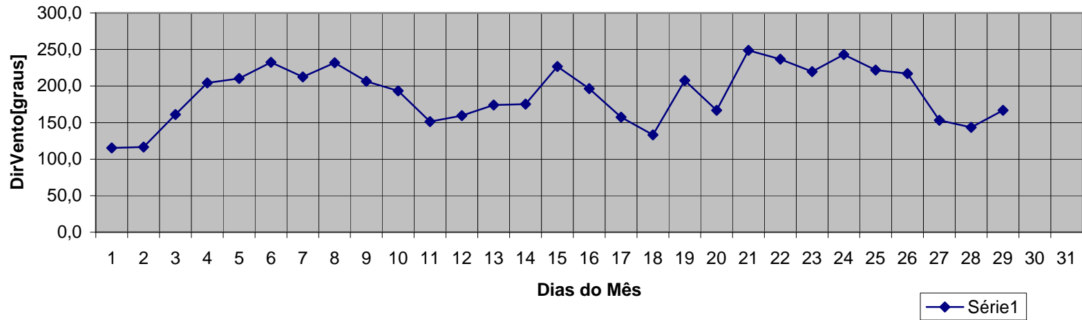
Média da direção do vento de maio_2008
