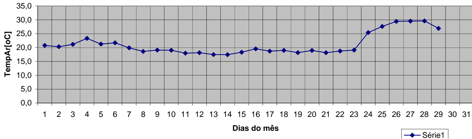
Média da temperatura de maio_2008
