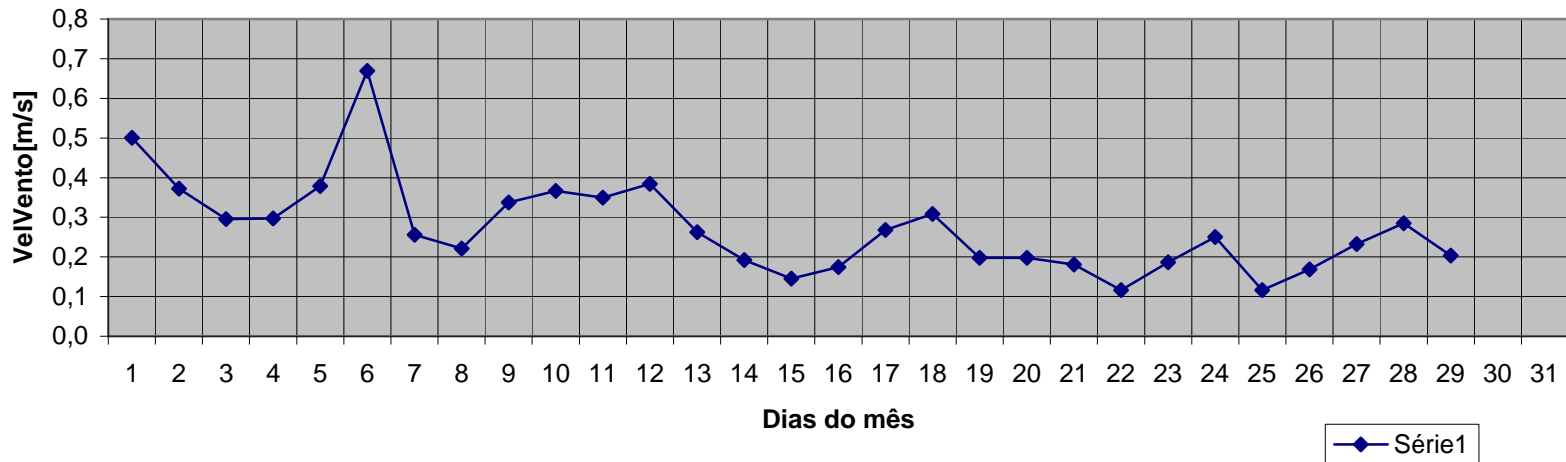
Média da velocidade do vento de maio_2008
