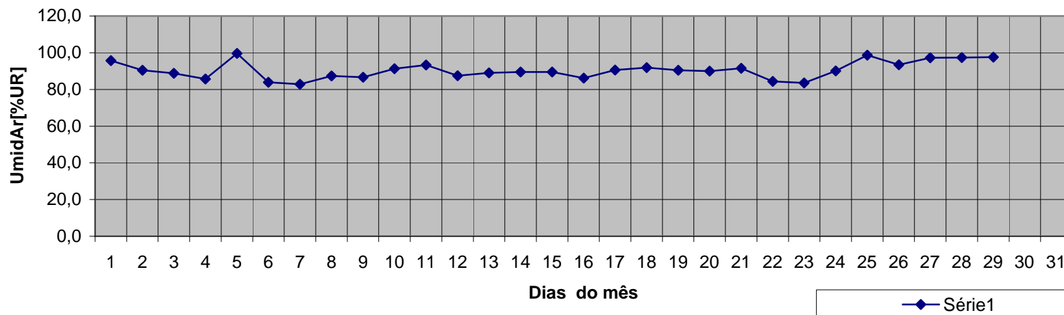
Média da umidade relativa do ar de maio_2008
